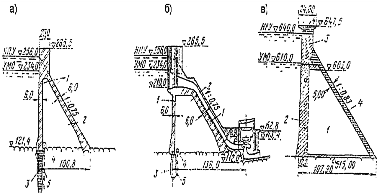
Расми 3. Намудҳои сарбандҳои гравитатсионӣ аз бетони шиббакардашуда (УКБ)
