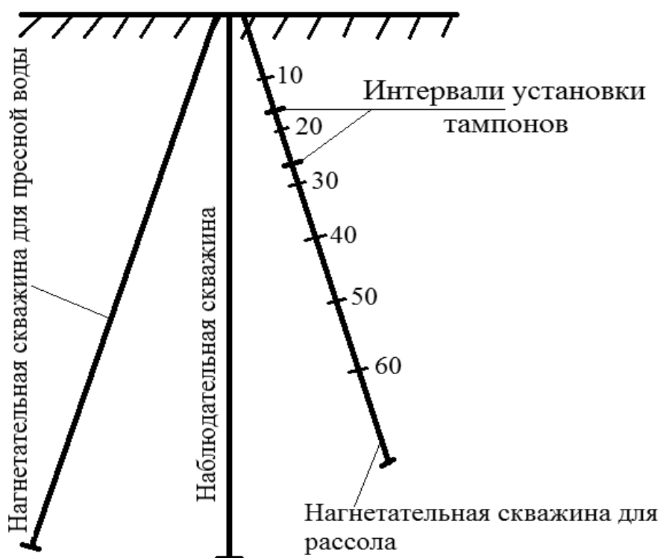
Рис. 2. Разрез куста скважин в опытной солевой камере
