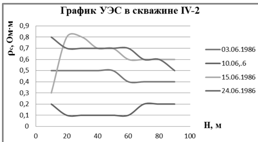
Рис. 4. График удельного электросопротивления минерализованных вод в скважине IV-2
