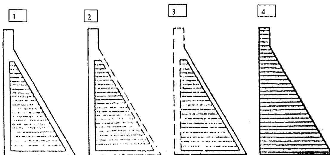
Расми 2. Намунаи сарбандҳо бо ядроӣ аз бетони шиббакардашуда
