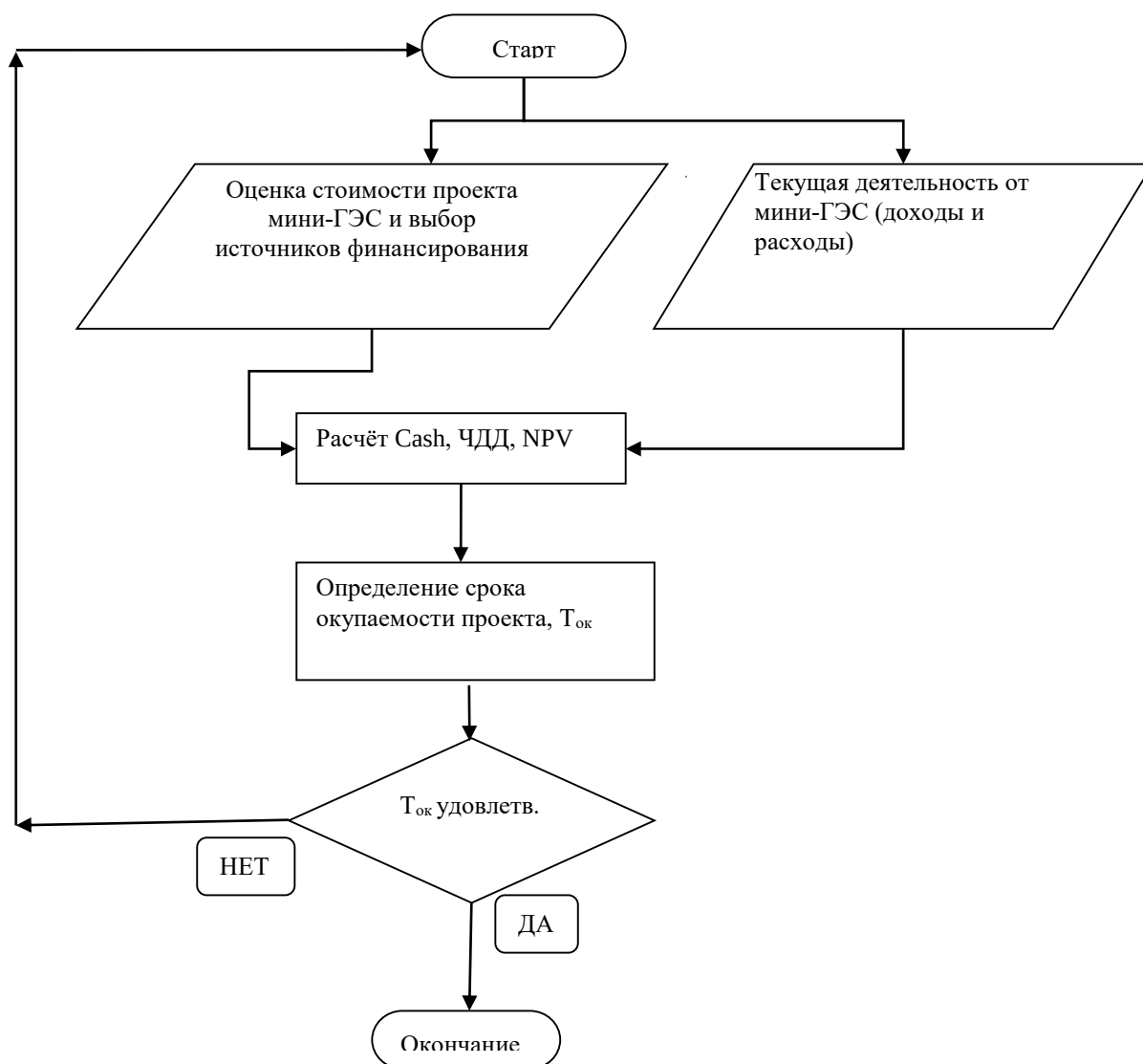
Рисунок 1. Алгоритм оценки эффективности реализации проекта мини-ГЭС.
