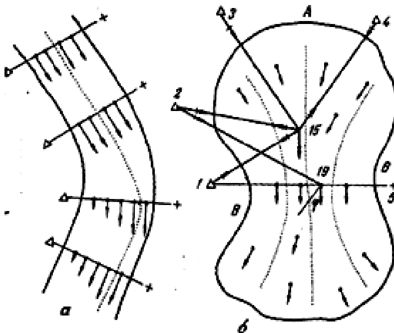
Рис. 2. Типы смещений: а) - земляной поток; б) - вращательный оползень; 1- опорный репер; 2 - ориентирный знак; 3 - оползневая точка; 4 - вектор смещения; 5 - траектории движения; 6 - направление визирного луча.
