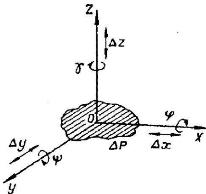
Рис. 3. Элементы движение на склоне
