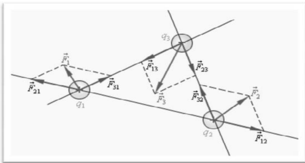
Расми 1. Принципи суперпозитсияи қувваҳои электростатикӣ
