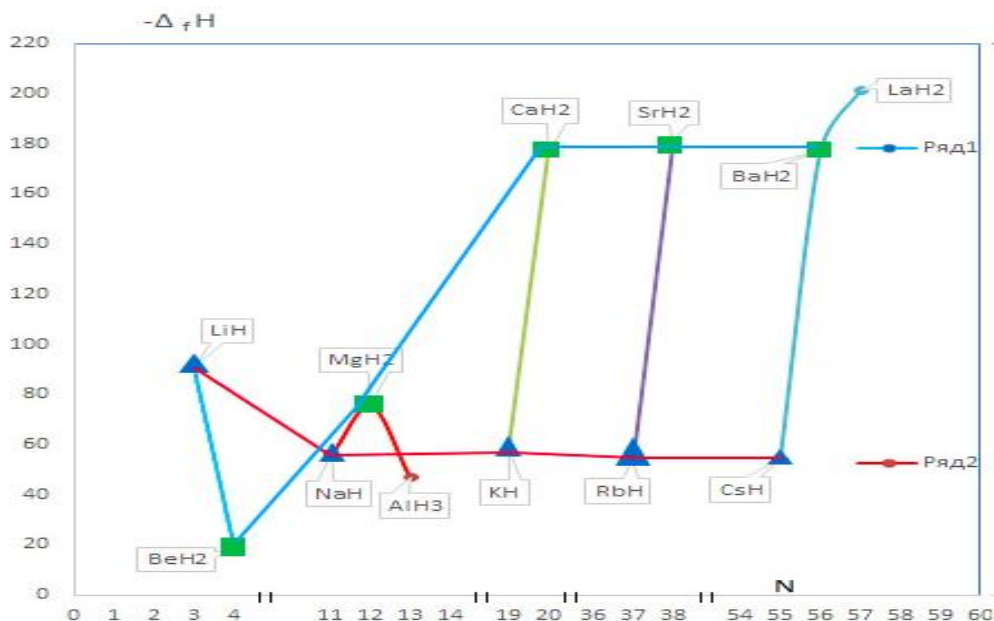
Рисунок 3. Графики изменения энтальпии образования бинарных гидридов в зависимости от природы катионов в периодах.
