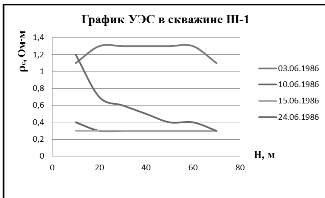
Рис. 7. График удельного электросопротивления минерализованных вод в скважине III-1
