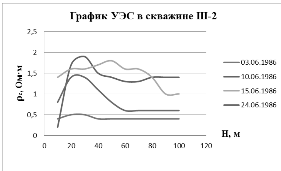
Рис. 5. График удельного электросопротивления минерализованных вод в скважине III-2
