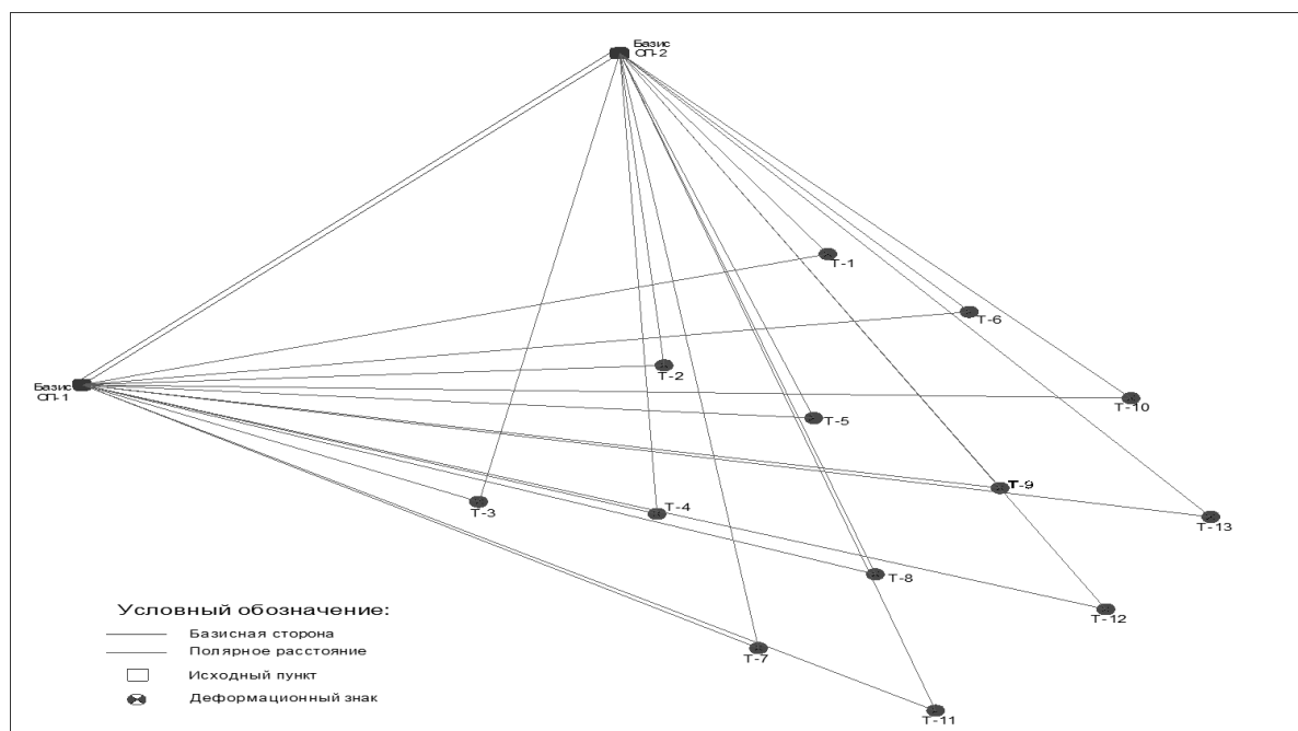
Рис. 8. Схема линейно-угловых измерений, определения координат исходных деформационных знаков в масштабе 1:1000
