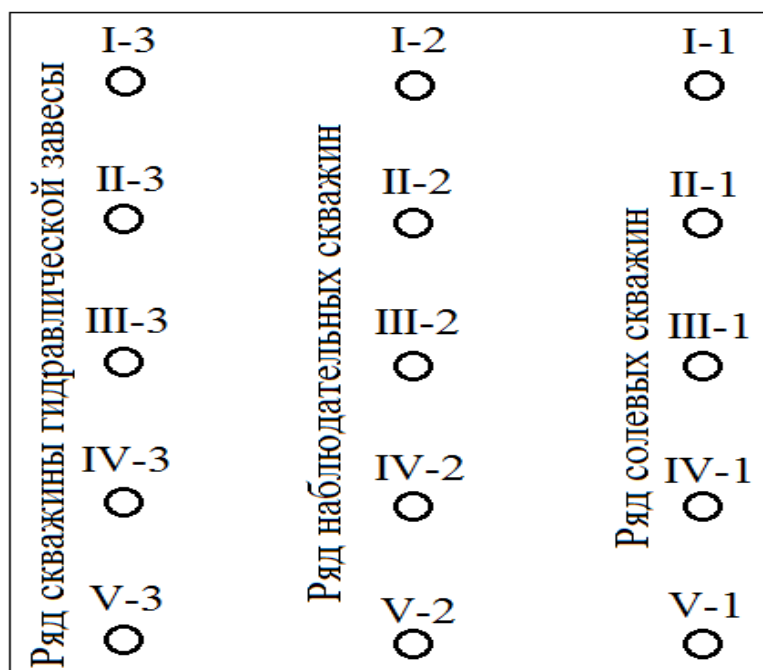
Рис. 1. План расположения скважин в опытной солевой камере
