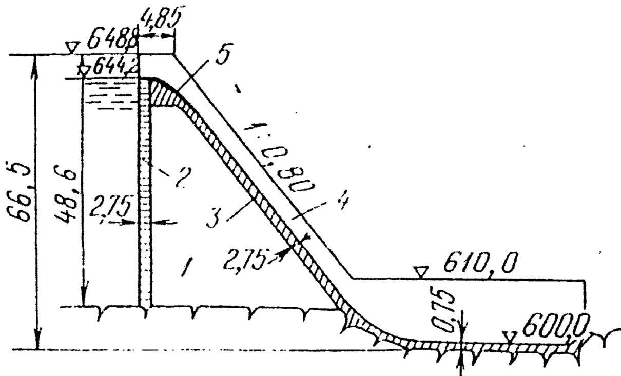
Расми 6. Сарбанди Уиллоу-Крик
