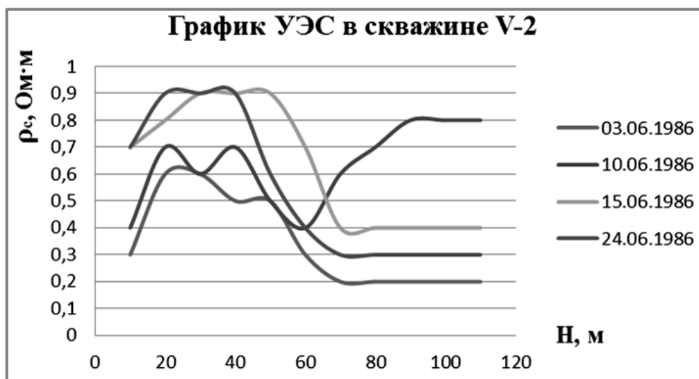
Рис. 3. График удельного электросопротивления минерализованных вод в скважине V-2
