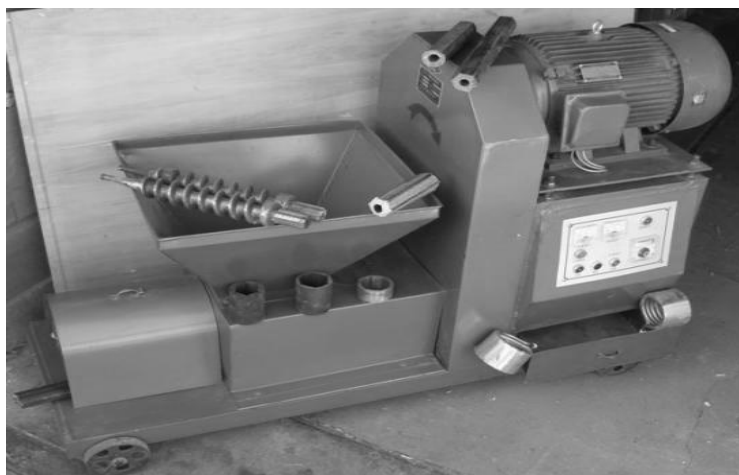
Рисунок 3 – Шнековый пресс
