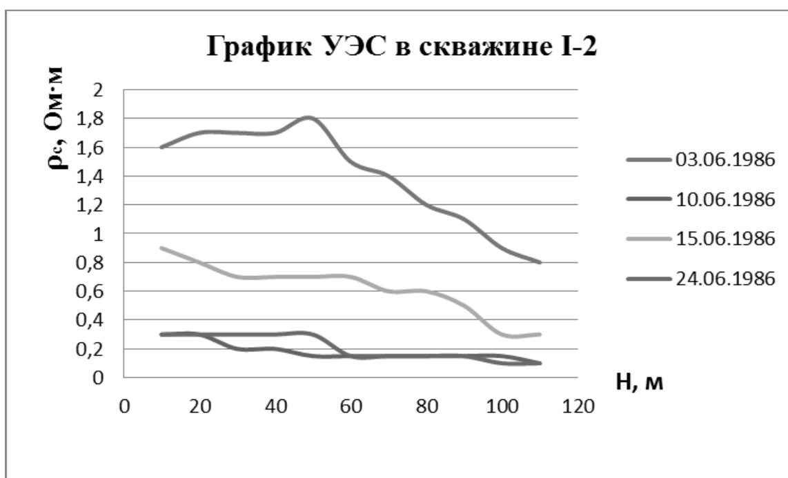
Рис. 6. График удельного электросопротивления минерализованных вод в скважине I-2
