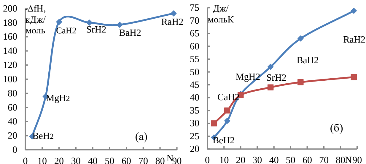
Рисунок 1. Графики зависимости энтальпии (а), энтропии (б) и теплоёмкости (б) образования бинарных гидридов IIIA от природы (N) катионов.
