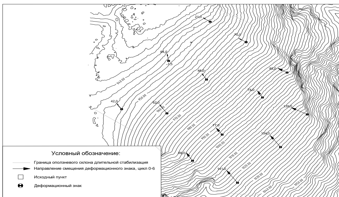
Рис. 7. Схема расположения одного из створов с деформационными знаками и данными, нанесенными в виде векторов, смещений оползневого тела за цикл между циклами наблюдений 0-6 в масштабе 1:1000
